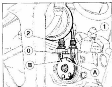
1) Élément de réglage / Einstellschraube / Registro 0) Indice "x" sur le couvercle / Indexgröße am Deckel / Índice fijo / tapa A) Indices sur la poulie / Anzeiger der Scheibe / Índice s/polea
